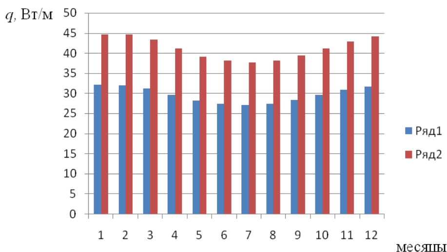
Рис. 4. – Результаты расчета удельных тепловых потерь паропровода d-76 мм. Ряд 1 – удельные тепловые потери без учета температурной деструкции ППУ-изоляции. Ряд 2 – удельные тепловые потери при увеличении коэффициента теплопроводности вследствие температурной деструкции на 20%
